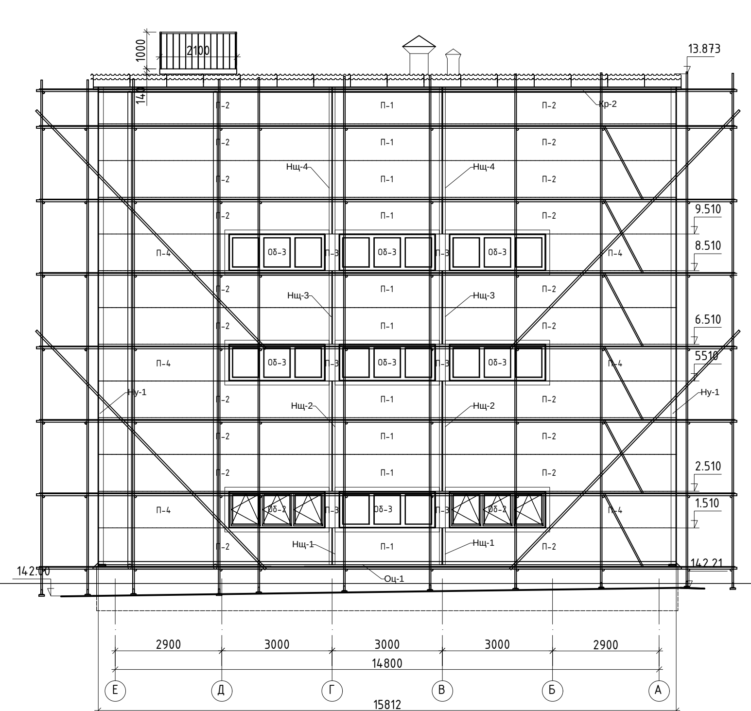
Западный фасад (в осях Е-А) М 1:100
