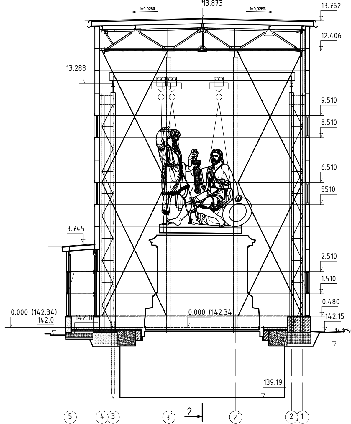
Разрез 1-1 М 1:100
