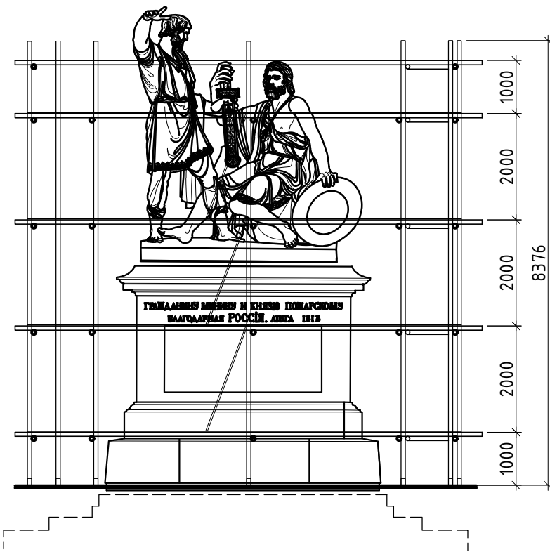
Схема установки лесов внутри павильона М 1:100
