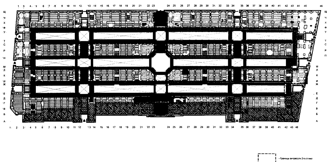
ПЛАН 2-ГО ЭТАЖА И АНТРЕСОЛИ 2-ГО ЭТАЖА
