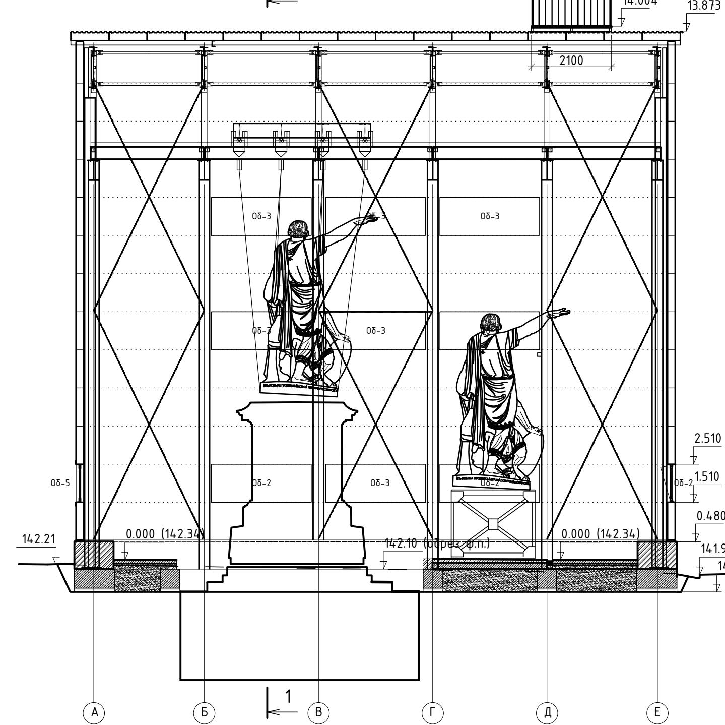
Разрез 2-2 М 1:100
