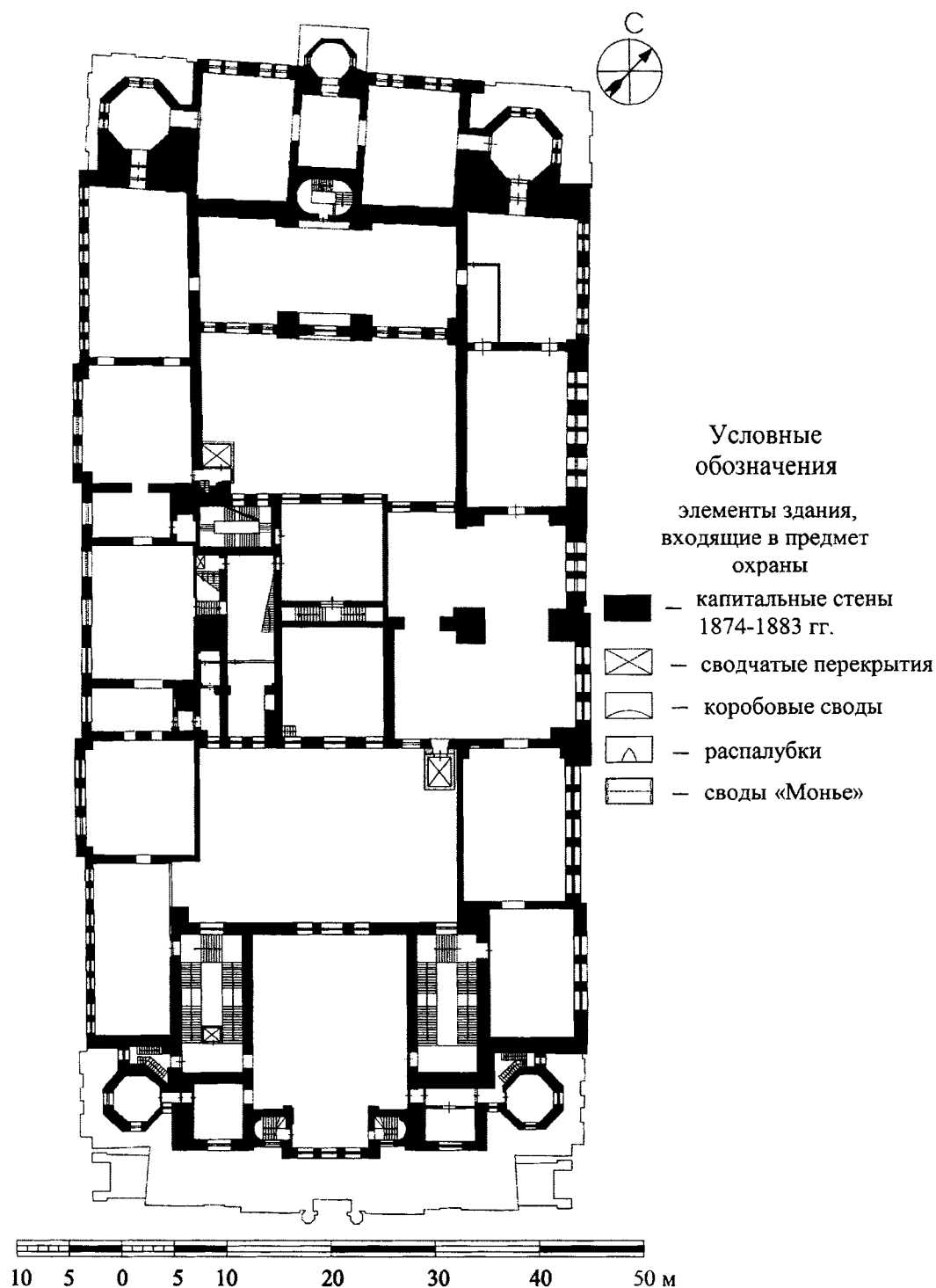
ПЛАН 3-ГО ЭТАЖА
