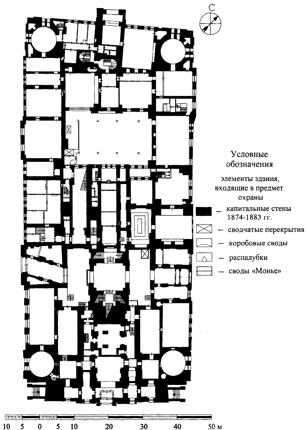
ПЛАН 1-ГО ЭТАЖА
