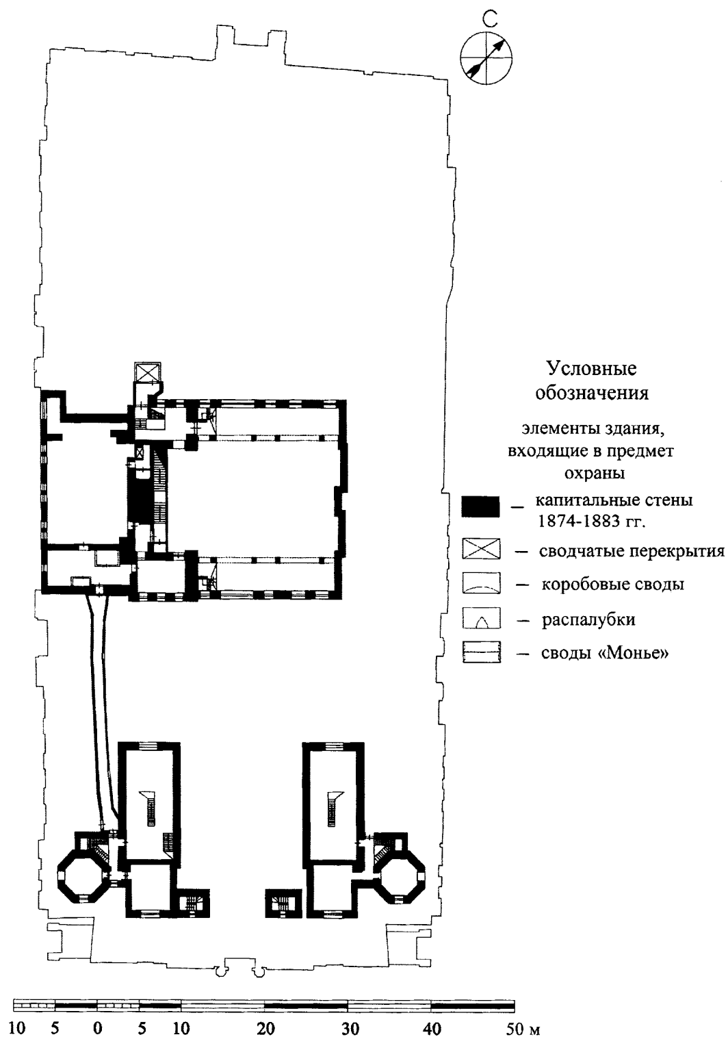
ПЛАН 4-ГО ЭТАЖА
