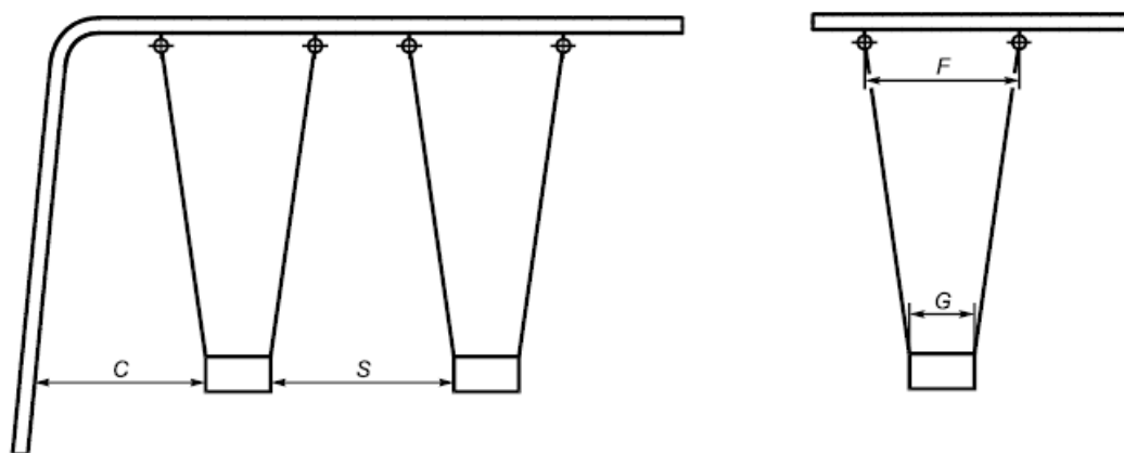
а) Минимальные расстояния между сиденьями качелей и смежной конструкцией
