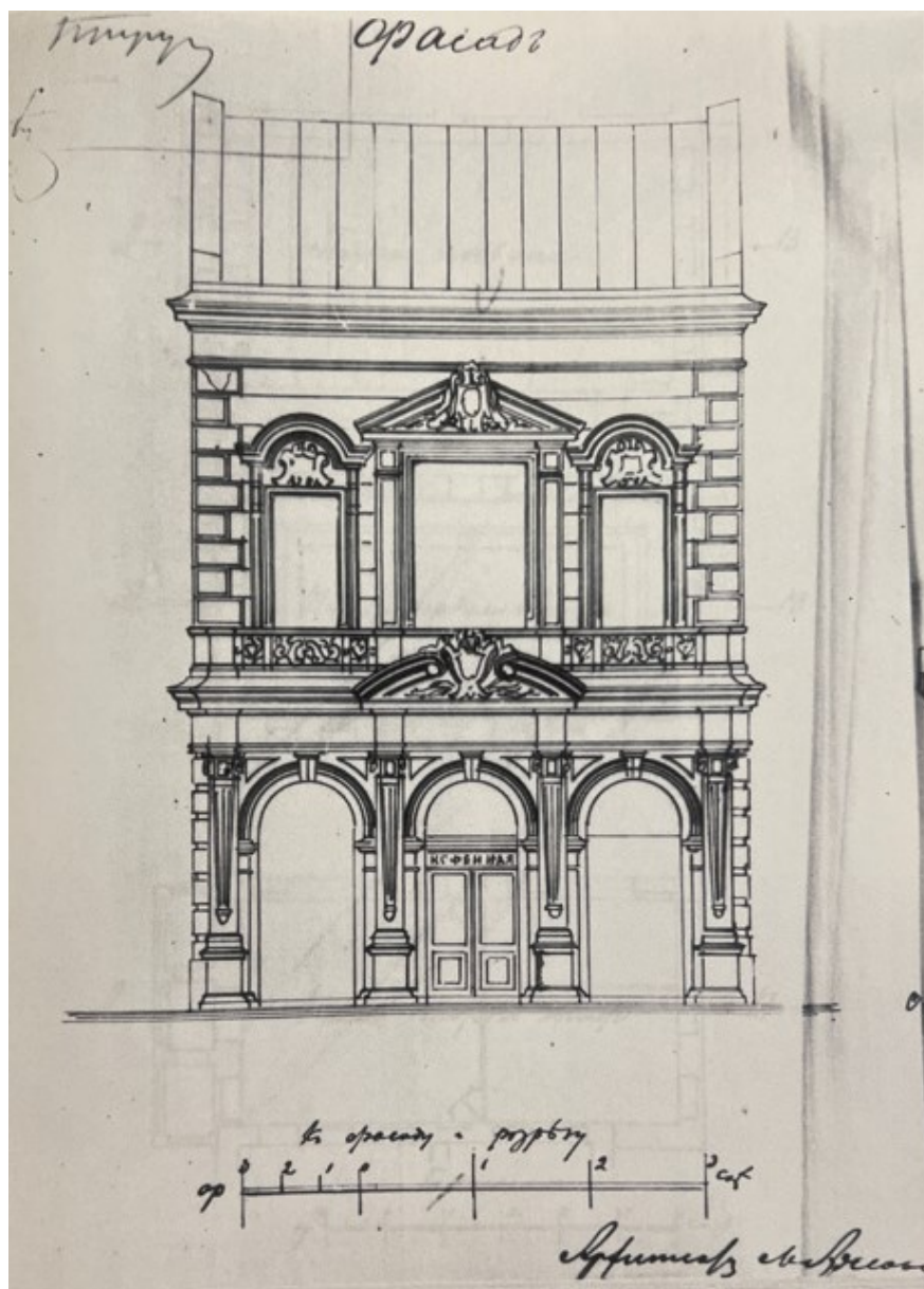
33. Фасад пристройки по Тверской ул. во владении Д. И. Филиппова. Архитектор М. А. Арсеньев. Июль 1885 г. Местоположение: ЦАНТДМ, ф. 1, Тверская часть, № 410/440, д. 12, л. 5. Источник: Историко-архитектурные исследования исторического домовладения по адресу Тверская улица, 10, стр. 1, 2, 3, 4 (квартал № 67). Альбом № 2. / Центр историко-градостроительных исследований. – Москва, 2004. – С. 77.
