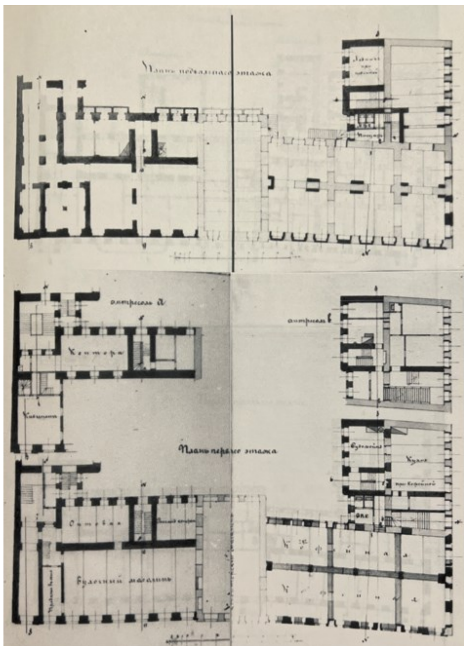
43. Поэтажные планы строения под №1 во владении Д. И. Филиппова. Архитектор М. А. Арсеньев. 1892 г. Местоположение: ЦАНТДМ, ф. 1, Тверская часть, № 410/440, д. 22, л. 9. Источник: Историко-архитектурные исследования исторического домовладения по адресу Тверская улица, 10, стр. 1, 2, 3, 4 (квартал № 67). Альбом № 2. / Центр историко-градостроительных исследований. – Москва, 2004. – С. 101.
