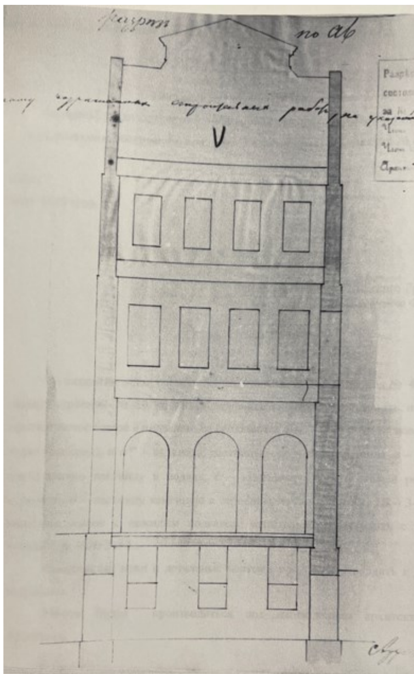
37. Разрез пристройки по Тверской ул. во владении Д. И. Филиппова. Архитектор М. А. Арсеньев. Август-сентябрь 1885 г. Местоположение: ЦАНТДМ, ф. 1, Тверская часть, № 410/440, д. 13, л. 11. Источник: Историко-архитектурные исследования исторического домовладения по адресу Тверская улица, 10, стр. 1, 2, 3, 4 (квартал № 67). Альбом № 2. / Центр историко-градостроительных исследований. – Москва, 2004. – С. 81.
