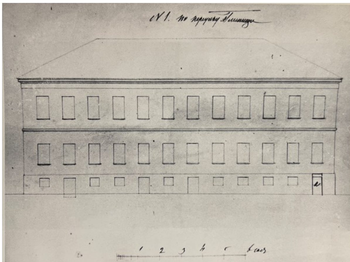
28. Фасад строения под № 1 по Глинищевскому пер. во владении жены подпоручика Ю. Д. Манухиной. 1862 г. Местоположение: ЦАНТДМ, ф. 1, Тверская часть, № 410/440, д. 5. Источник: Историко-архитектурные исследования исторического домовладения по адресу Тверская улица, 10, стр. 1, 2, 3, 4 (квартал № 67). Альбом № 2. / Центр историко-градостроительных исследований. – Москва, 2004. – С. 65.
