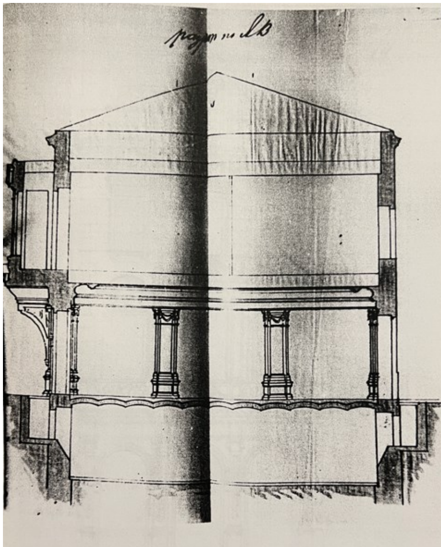
35. Разрез пристройки по Тверской ул. во владении Д. И. Филиппова. Архитектор М. А. Арсеньев. Июль 1885 г. Местоположение: ЦАНТДМ, ф. 1, Тверская часть, № 410/440, д. 12, л. 5. Источник: Историко-архитектурные исследования исторического домовладения по адресу Тверская улица, 10, стр. 1, 2, 3, 4 (квартал № 67). Альбом № 2. / Центр историко-градостроительных исследований. – Москва, 2004. – С. 79.
