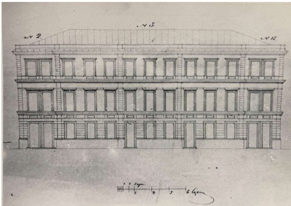
26. Фасад строений под № 2, 3, 13 по Тверской ул. во владении наследников Поповых. 1859 г. Местоположение: ЦАНТДМ, ф. 1, Тверская часть, № 410/440, д. 5. Источник: Историко-архитектурные исследования исторического домовладения по адресу Тверская улица, 10, стр. 1, 2, 3, 4 (квартал № 67). Альбом № 2. / Центр историко-градостроительных исследований. – Москва, 2004. – С. 63.
