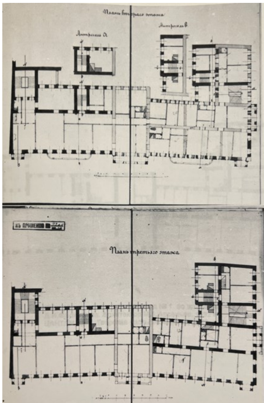
44. Поэтажные планы строения под №1 во владении Д. И. Филиппова. Архитектор М. А. Арсеньев. 1892 г. Местоположение: ЦАНТДМ, ф. 1, Тверская часть, № 410/440, д. 22, л. 9. Источник: Историко-архитектурные исследования исторического домовладения по адресу Тверская улица, 10, стр. 1, 2, 3, 4 (квартал № 67). Альбом № 2. / Центр историко-градостроительных исследований. – Москва, 2004. – С. 102.
