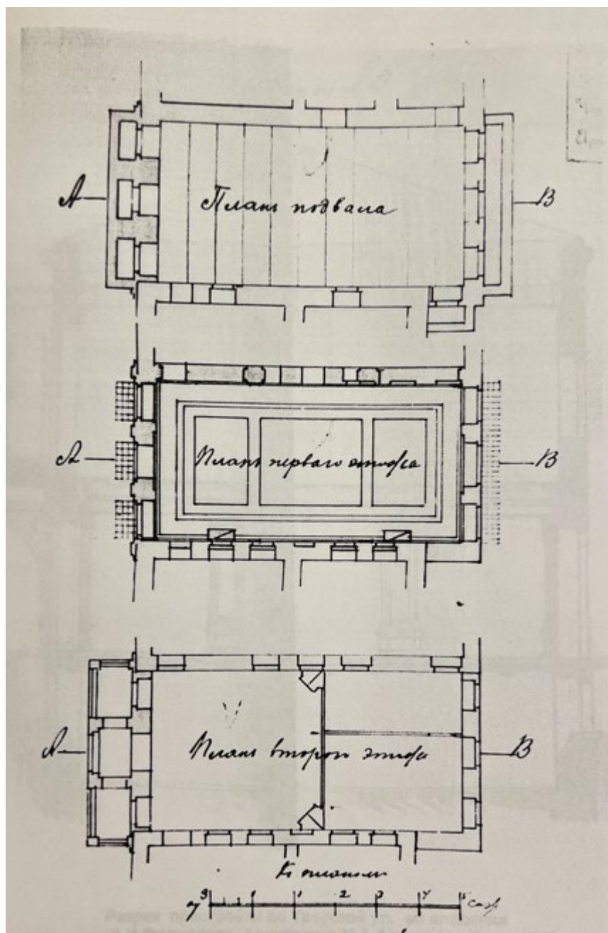
34. Поэтажные планы пристройки по Тверской ул. во владении Д. И. Филиппова. Архитектор М. А. Арсеньев. Июль 1885 г. Местоположение: ЦАНТДМ, ф. 1, Тверская часть, № 410/440, д. 12, л. 5. Источник: Историко-архитектурные исследования исторического домовладения по адресу Тверская улица, 10, стр. 1, 2, 3, 4 (квартал № 67). Альбом № 2. / Центр историко-градостроительных исследований. – Москва, 2004. – С. 78.
