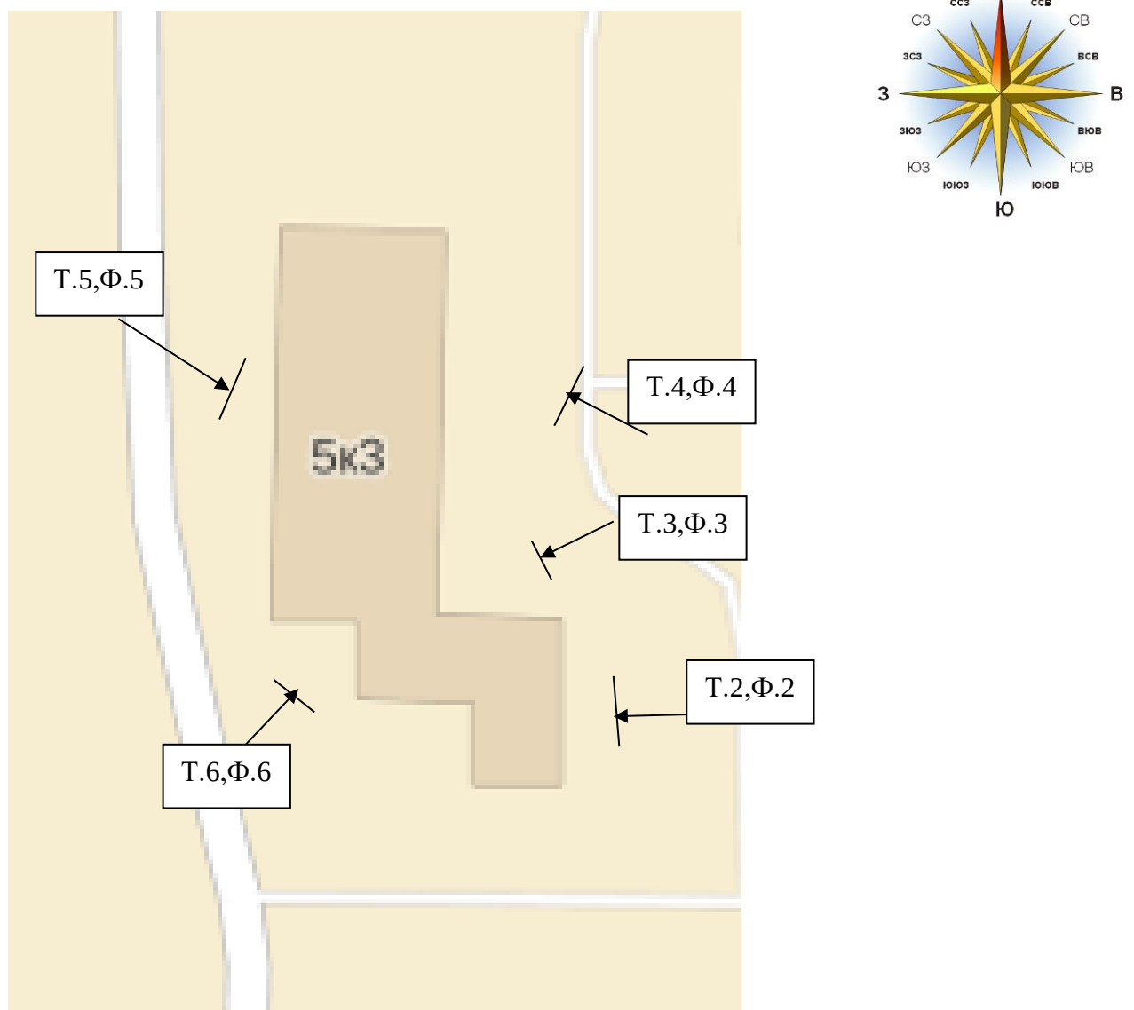
Рис. 2. Схема термографирования фасадов 3-ей Радиаторской ул., д.5, к.3
