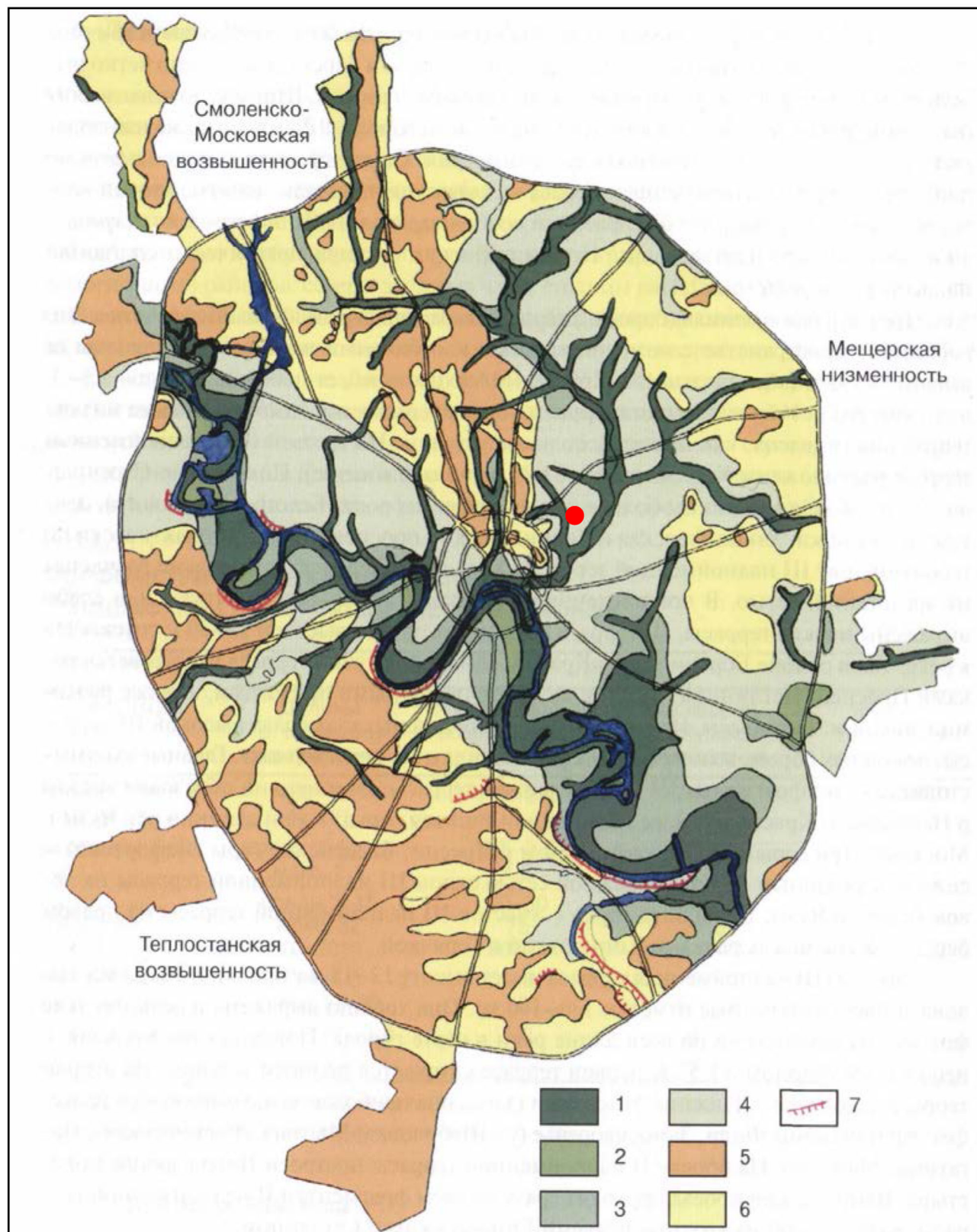
Илл. 4. Геоморфологическая схема с указанием основных элементов гидрографической сети г. Москвы. Фрагмент. Из кн.: Москва. Геология и город. М., 1997.
