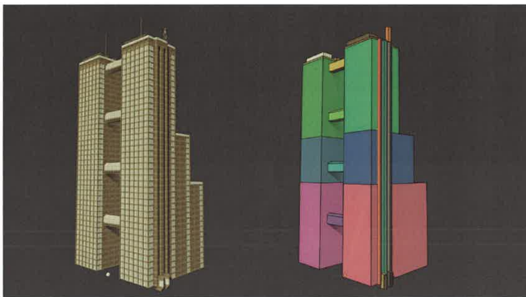
Рис. 7.1. Оригинальная модель и ее геометрия коллизии
